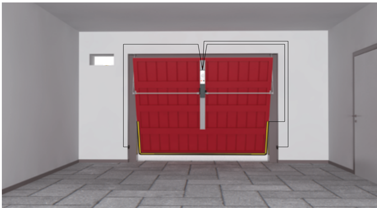
IMPIANTO TIPO CON MONTAGGIO CENTRALE
