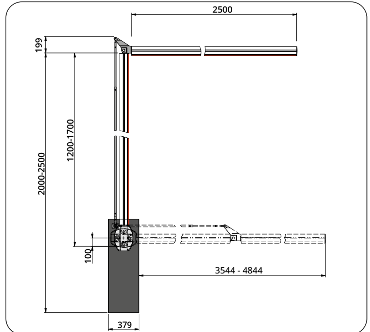
Snodo per asta ellittica
